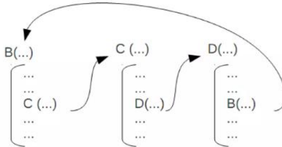
Récurtivité indirecte
