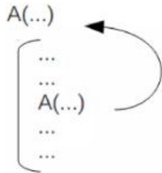
Récurtivité directe
